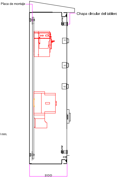
VISTA LATERAL
